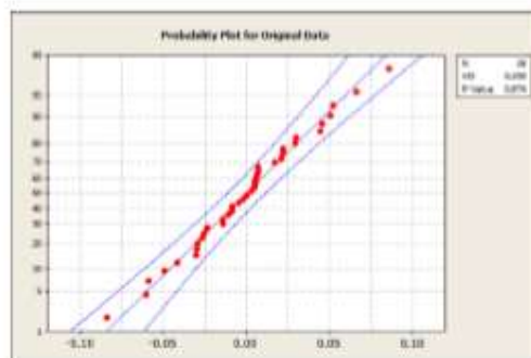
شکل ۴.۱: نمودار احتمال نرمال برای مدل رگرسیونی
