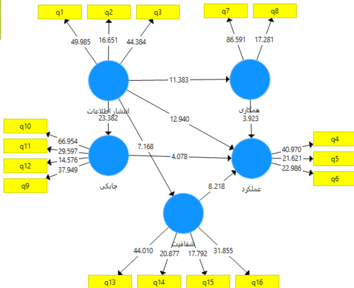
شکل ۳: معناداری مدل
